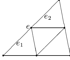
FIGURE 2. An edge e \in \mathcal{E}_{k-1} .
